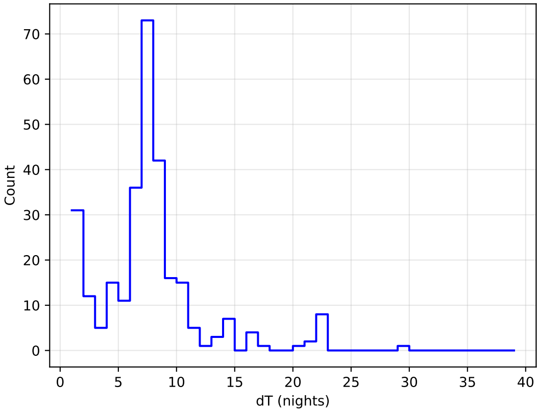
no_magell_roll_v3.4_10yrs all bands: DD:EDFS Delta Nights Histogram
