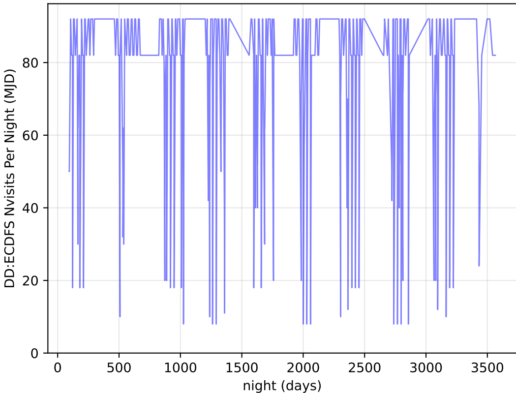
no_magell_roll_v3.4_10yrs all bands: DD:ECDFS Nvisits Per Night
