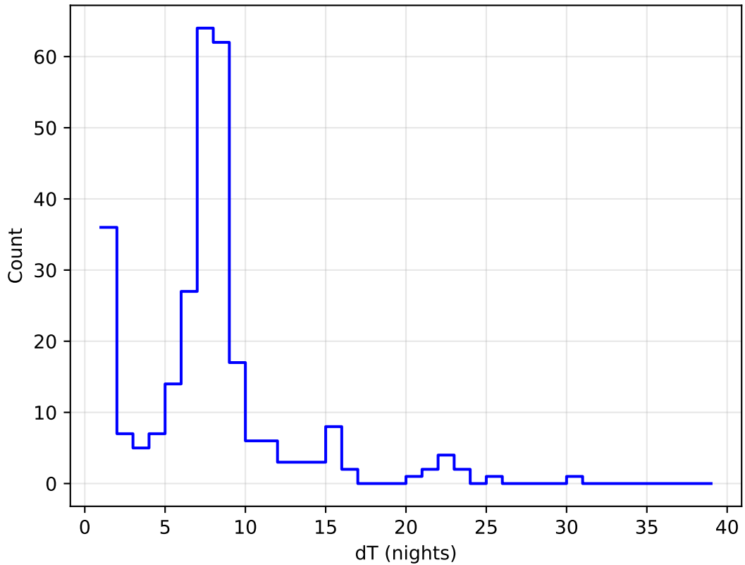
no_magell_roll_v3.4_10yrs all bands: DD:ECDFS Delta Nights Histogram
