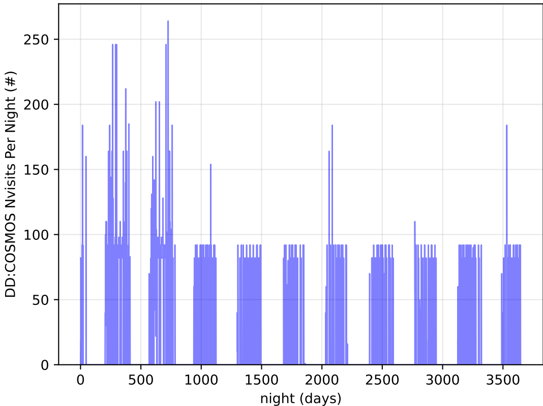
no_magell_roll_v3.4_10yrs all bands: DD: COSMOS Nvisits Per Night
