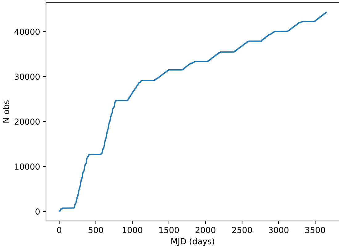
no_magell_roll_v3.4_10yrs all bands: DD:COSMOS Cumulative NVisits
