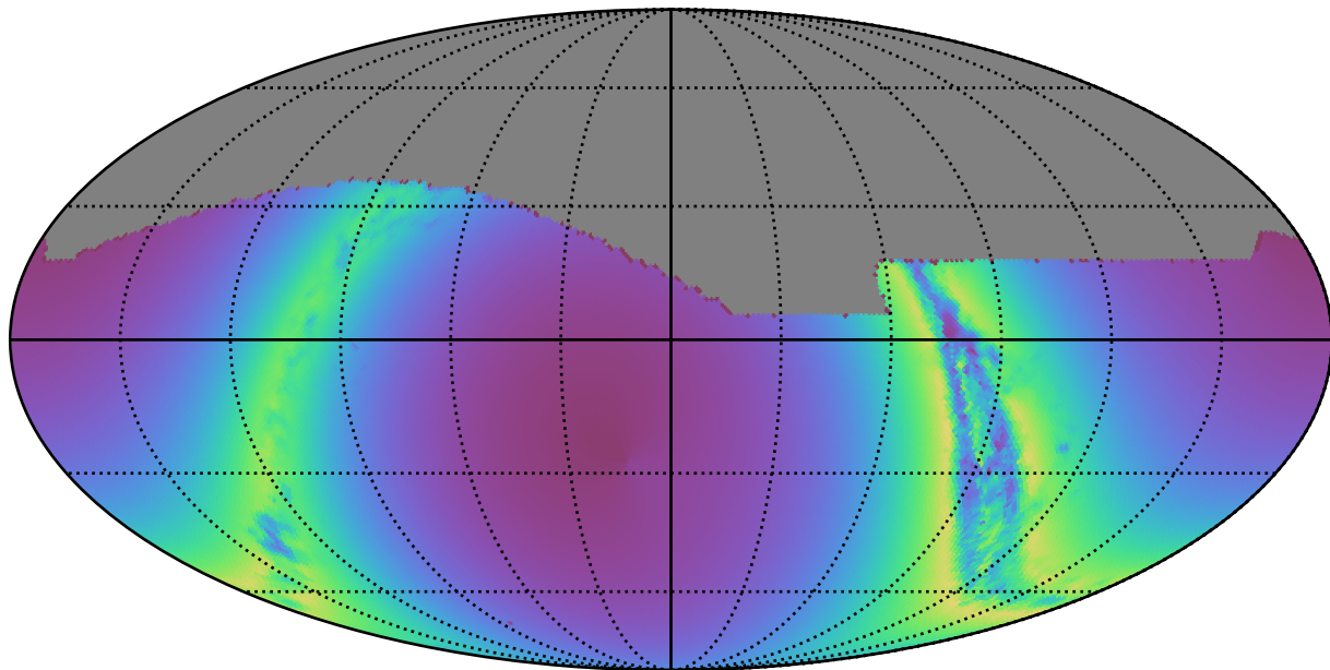
no_long_v3.4_10yrs : young_stars
