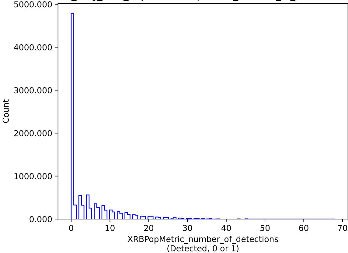
no_long_v3.4_10yrs : XRBPopMetric_number_of_detections
