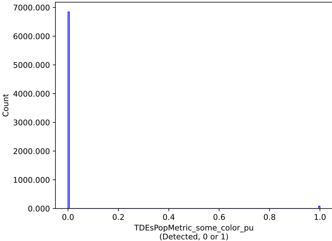
no_long_v3.4_10yrs : TDEsPopMetric_some_color_pu
