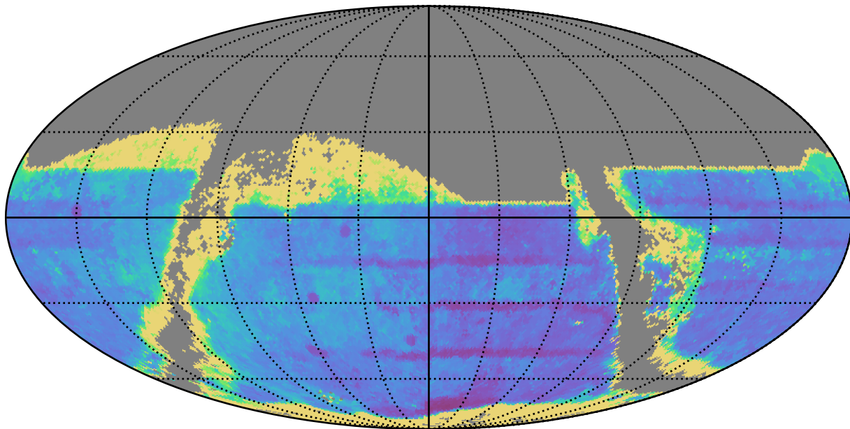
no_long_v3.4_10yrs : TDC_accuracy
