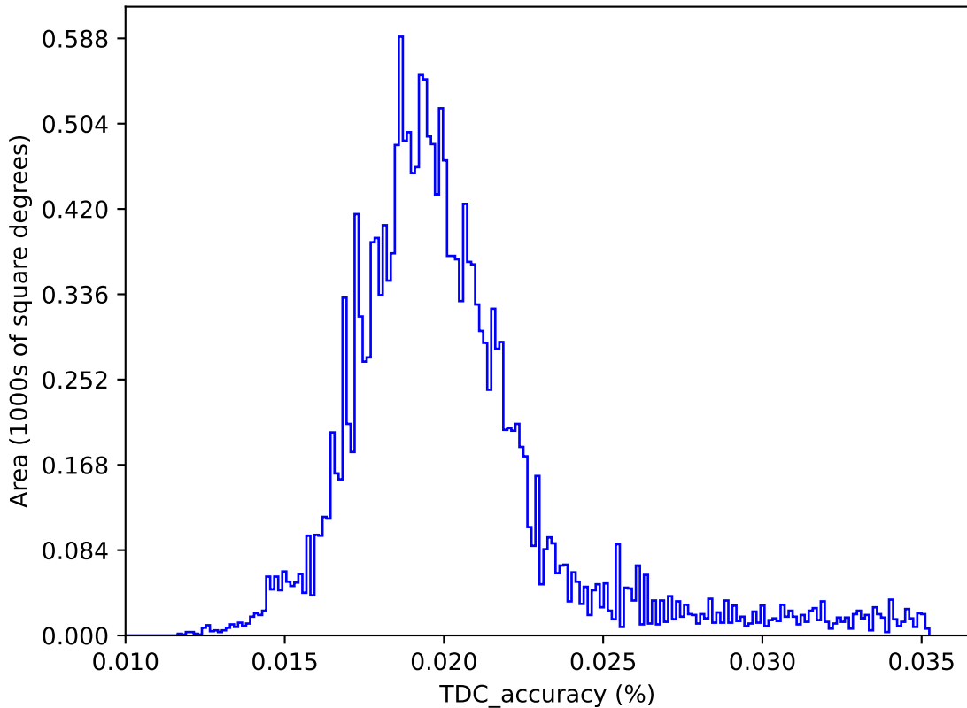
no_long_v3.4_10yrs : TDC_accuracy
