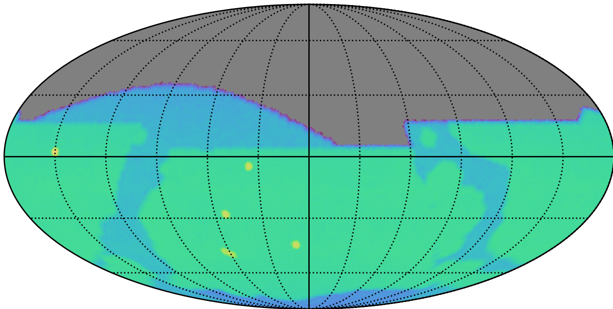
no_long_v3.4_10yrs i: SurfaceBrightLimit
