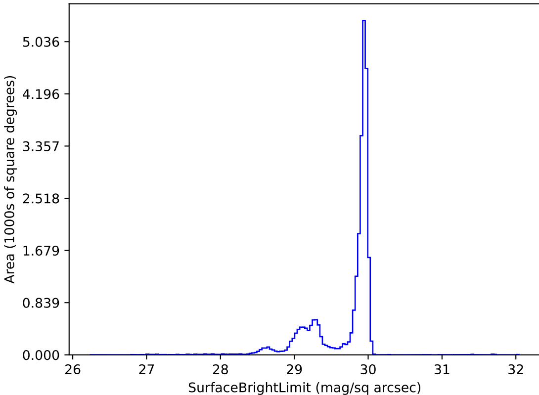
no_long_v3.4_10yrs i: SurfaceBrightLimit
