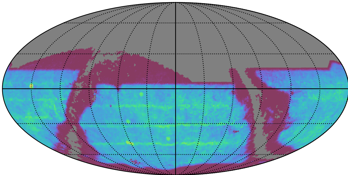
no_long_v3.4_10yrs : SNSLMetric
