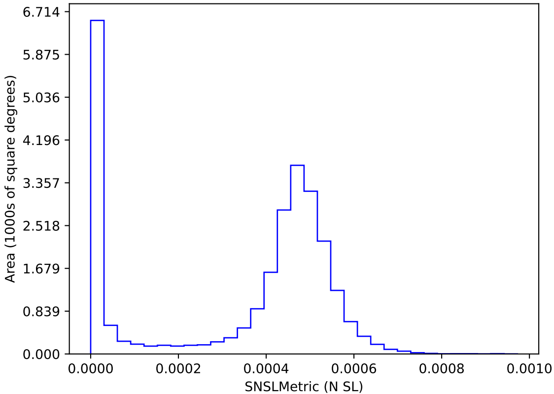
no_long_v3.4_10yrs : SNSLMetric
