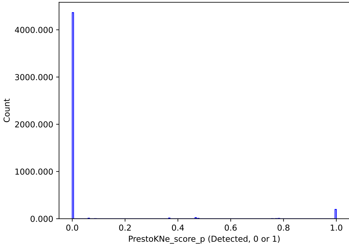
no_long_v3.4_10yrs : PrestoKNe_score_p
