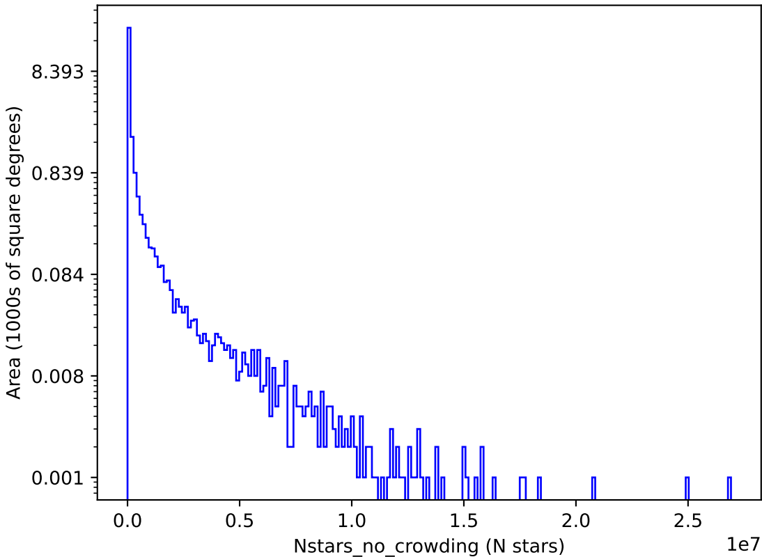
no_long_v3.4_10yrs z: Nstars_no_crowding
