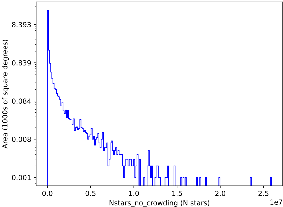
no_long_v3.4_10yrs y: Nstars_no_crowding
