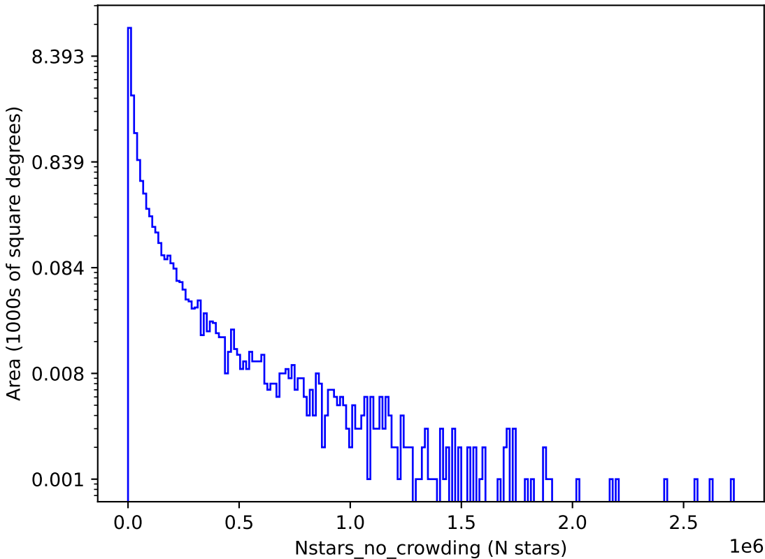
no_long_v3.4_10yrs u: Nstars_no_crowding
