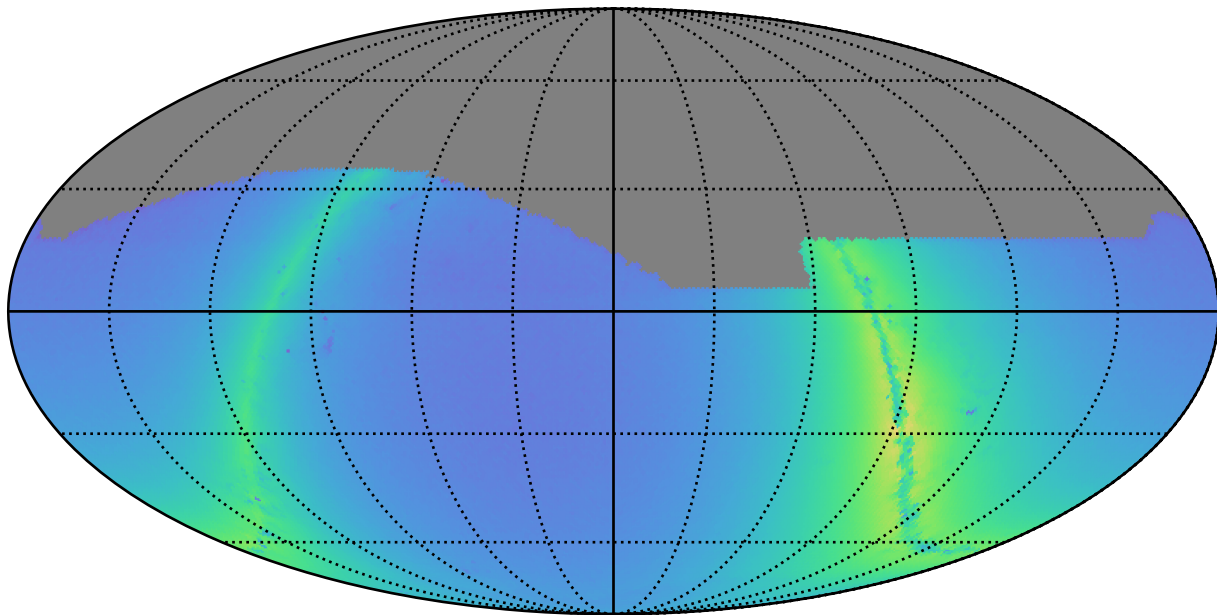
no_long_v3.4_10yrs i: Nstars_no_crowding
