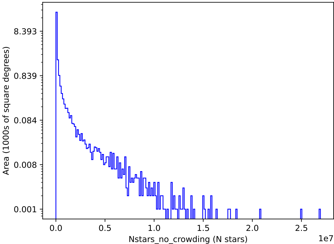
no_long_v3.4_10yrs i: Nstars_no_crowding
