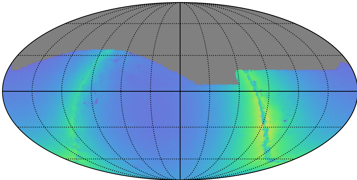
no_long_v3.4_10yrs g: Nstars_no_crowding
