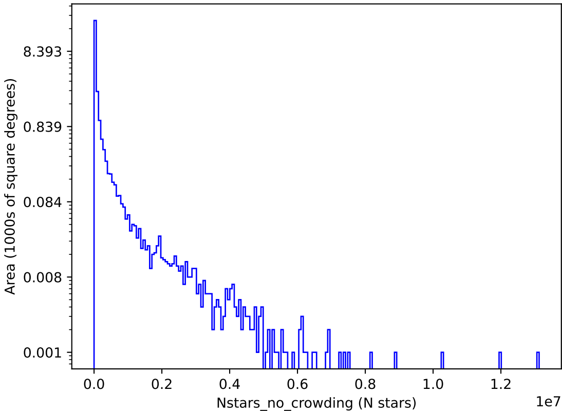
no_long_v3.4_10yrs g: Nstars_no_crowding
