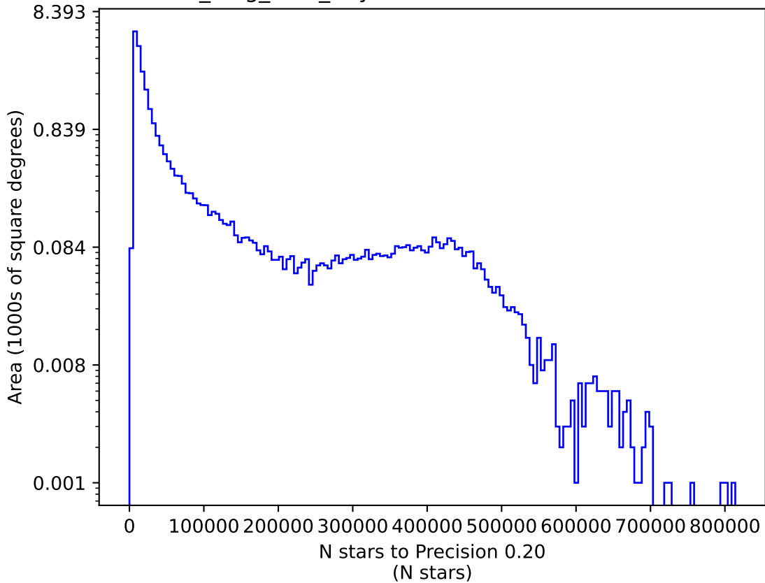
no_long_v3.4_10yrs i: N stars to Precision 0.20
