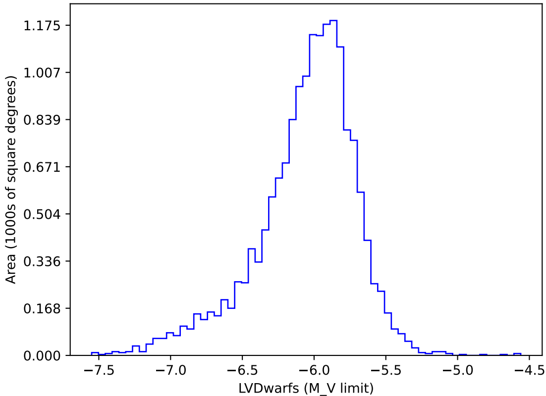
no_long_v3.4_10yrs gi: LVDwarfs
