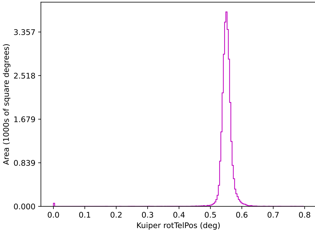
no_long_v3.4_10yrs z: Kuiper rotTelPos
