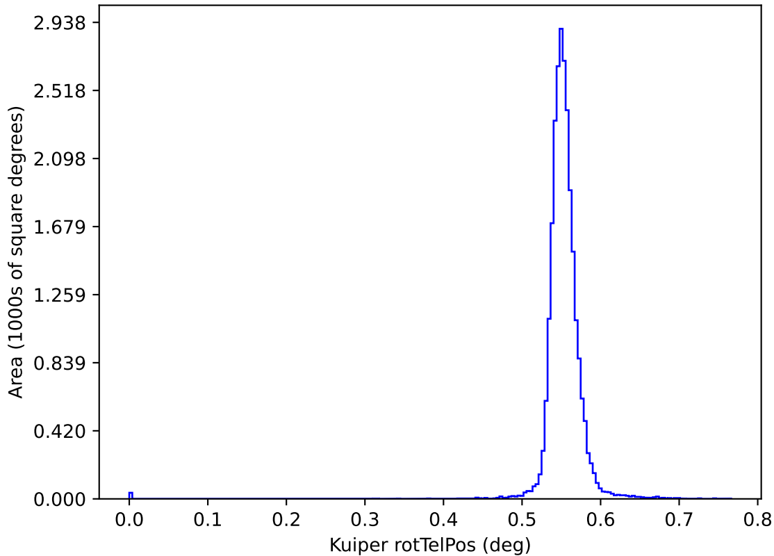
no_long_v3.4_10yrs y: Kuiper rotTelPos
