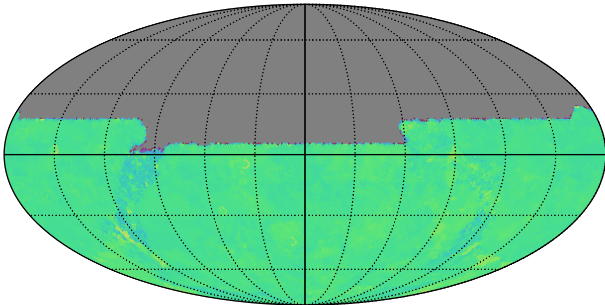
no_long_v3.4_10yrs u: Kuiper rotTelPos
