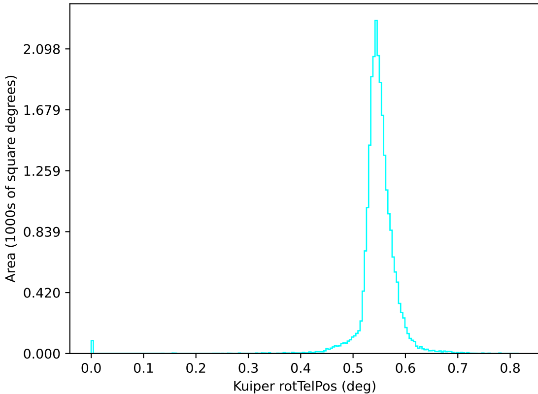
no_long_v3.4_10yrs u: Kuiper rotTelPos
