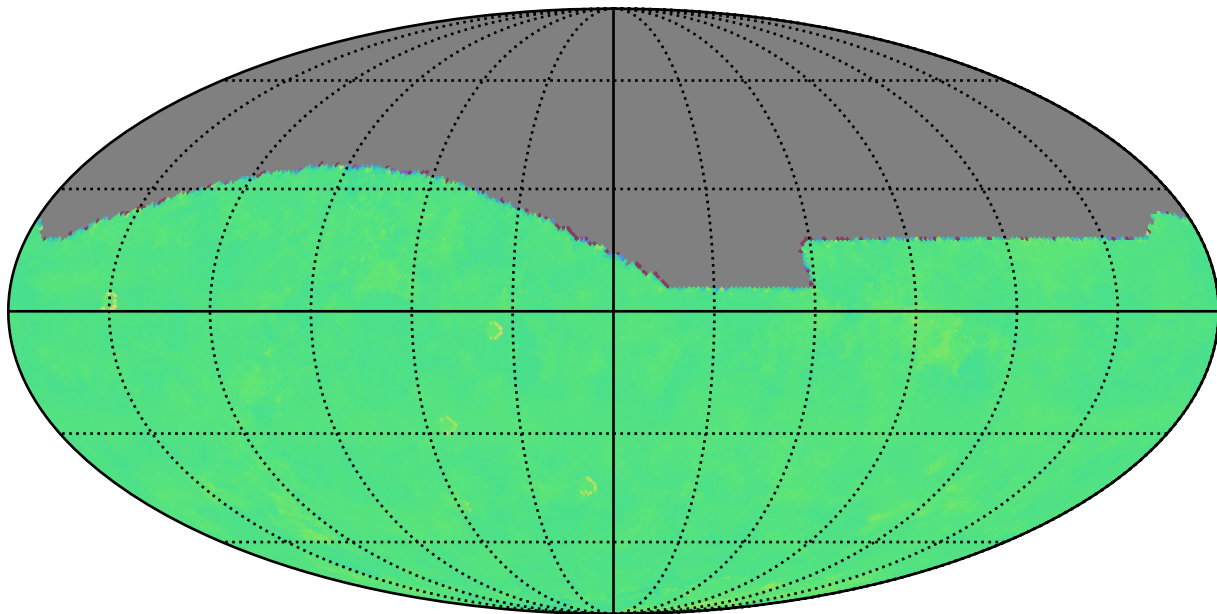
no_long_v3.4_10yrs i: Kuiper rotTelPos
