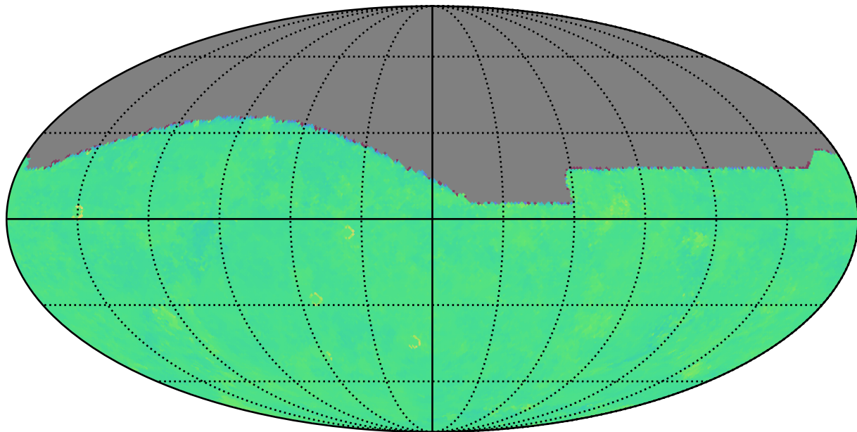
no_long_v3.4_10yrs g: Kuiper rotTelPos
