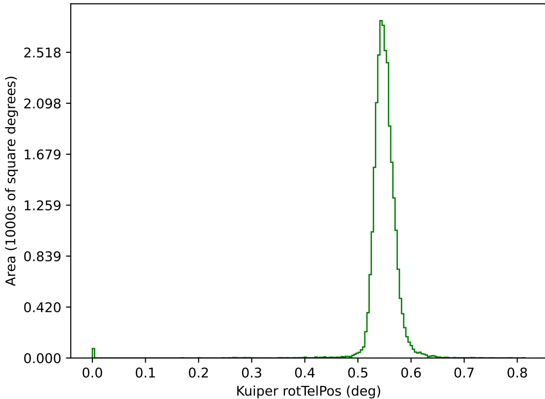
no_long_v3.4_10yrs g: Kuiper rotTelPos
