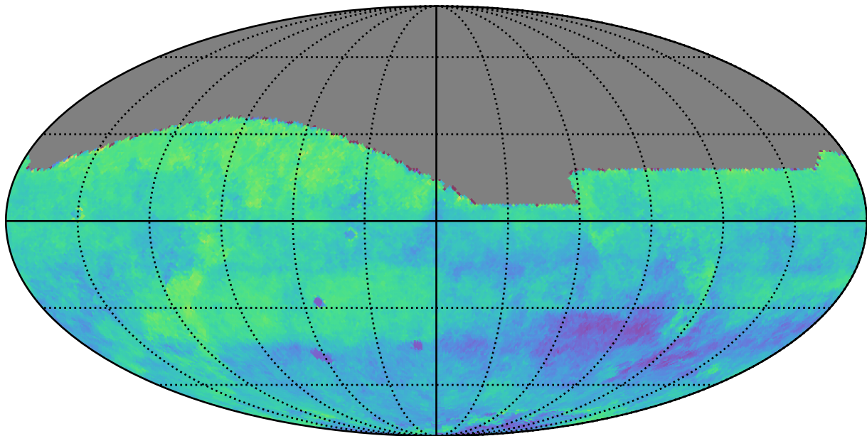
no_long_v3.4_10yrs z: Kuiper rotSkyPos
