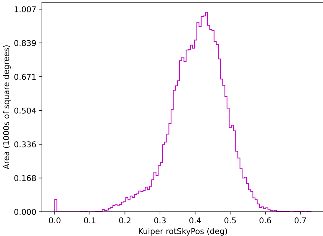
no_long_v3.4_10yrs z: Kuiper rotSkyPos
