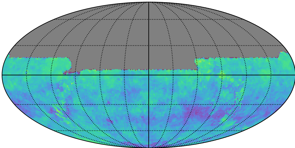
no_long_v3.4_10yrs u: Kuiper rotSkyPos
