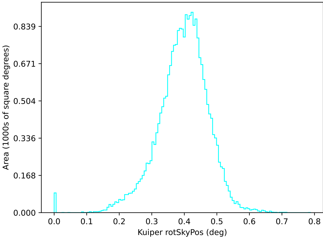
no_long_v3.4_10yrs u: Kuiper rotSkyPos
