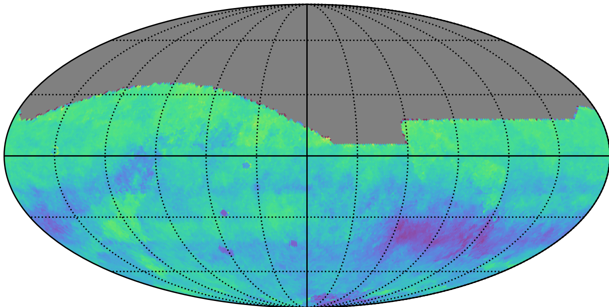
no_long_v3.4_10yrs r: Kuiper rotSkyPos
