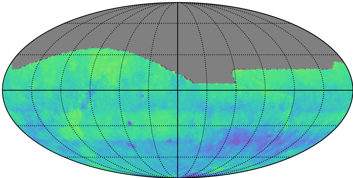
no_long_v3.4_10yrs i: Kuiper rotSkyPos
