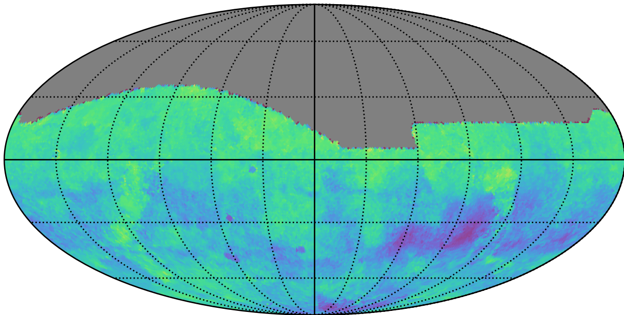
no_long_v3.4_10yrs g: Kuiper rotSkyPos
