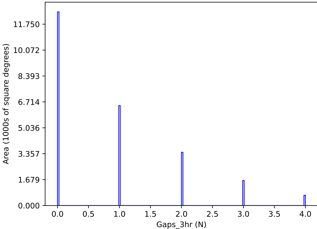
no_long_v3.4_10yrs y band: Gaps_3hr
