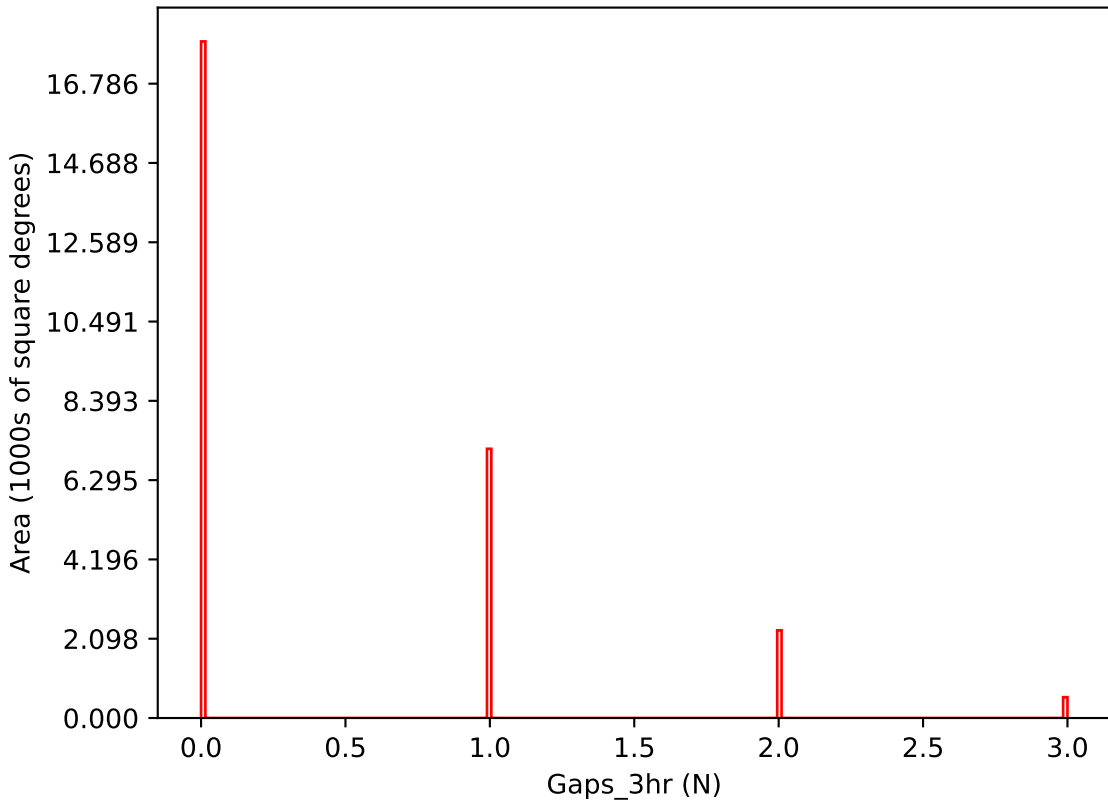
no_long_v3.4_10yrs i band: Gaps_3hr
