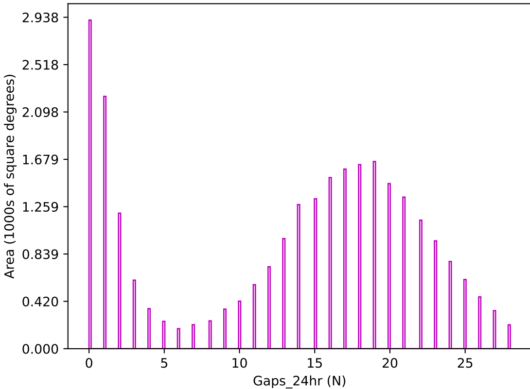
no_long_v3.4_10yrs z band: Gaps_24hr
