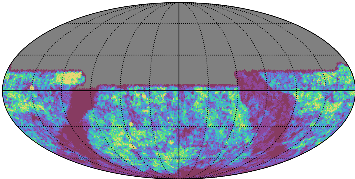
no_long_v3.4_10yrs u band: Gaps_24hr
