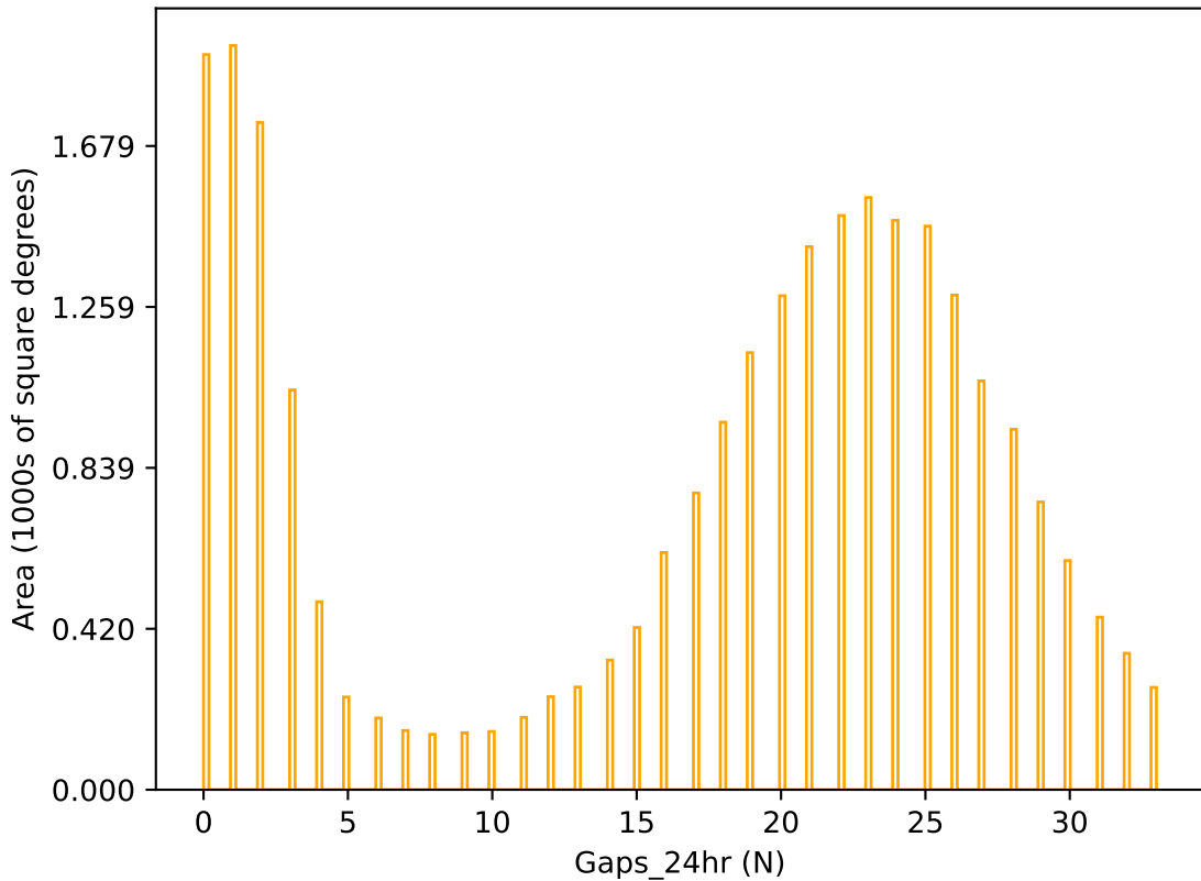
no_long_v3.4_10yrs r band: Gaps_24hr
