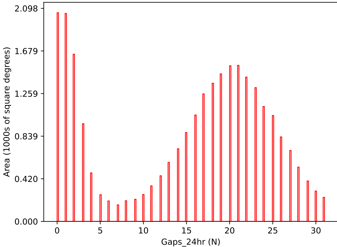
no_long_v3.4_10yrs i band: Gaps_24hr
