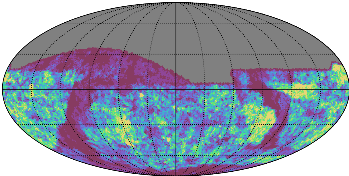
no_long_v3.4_10yrs g band: Gaps_24hr
