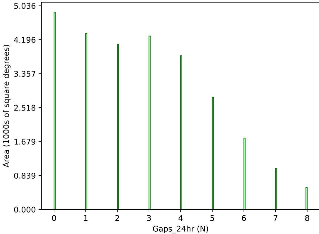
no_long_v3.4_10yrs g band: Gaps_24hr
