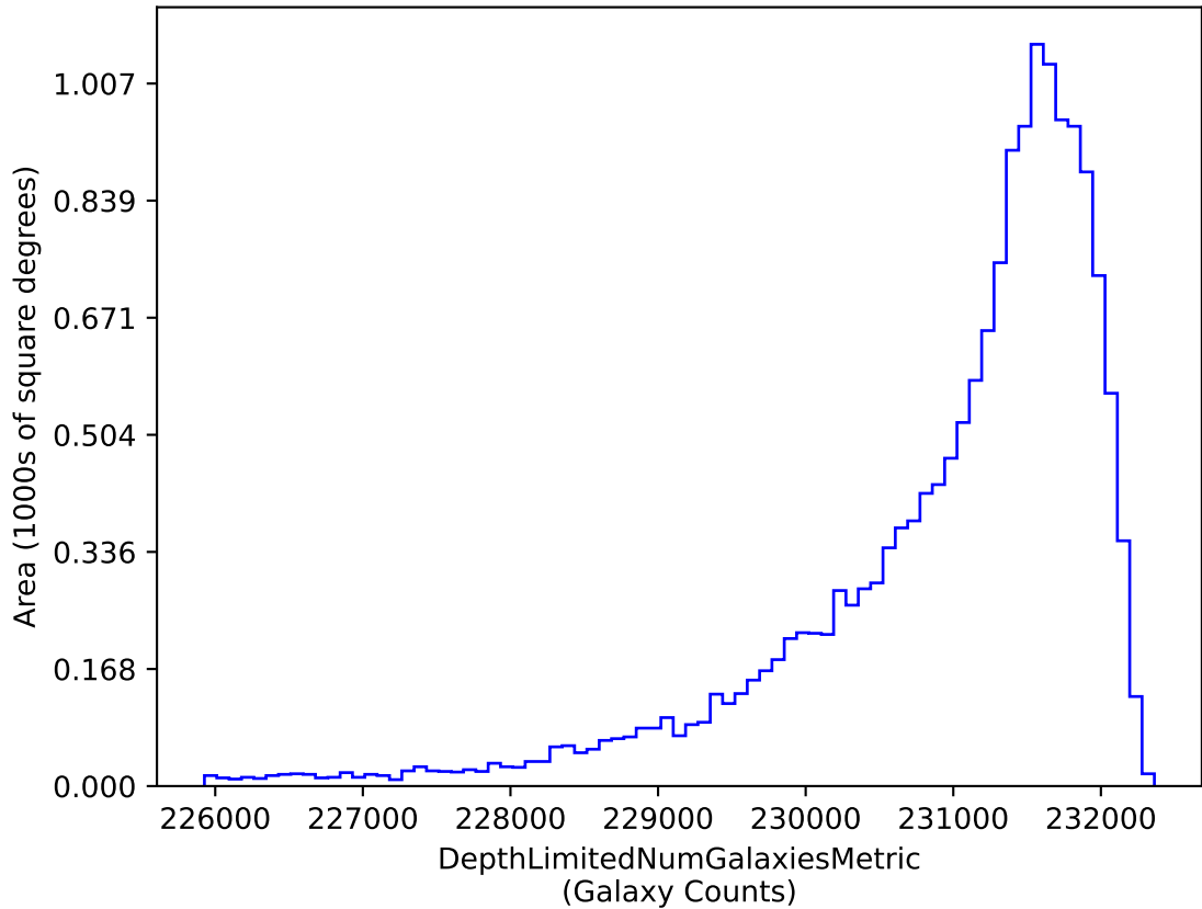
no_long_v3.4_10yrs i band galaxies non-DD: DepthLimitedNumGalaxiesMetric
