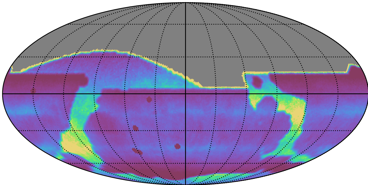
no_long_v3.4_10yrs : DCRprecision
