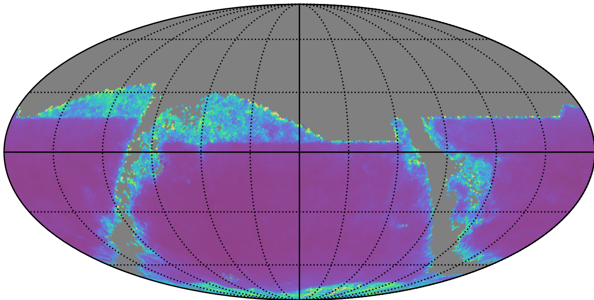
no_long_v3.4_10yrs z band: AGN SF_uncert
