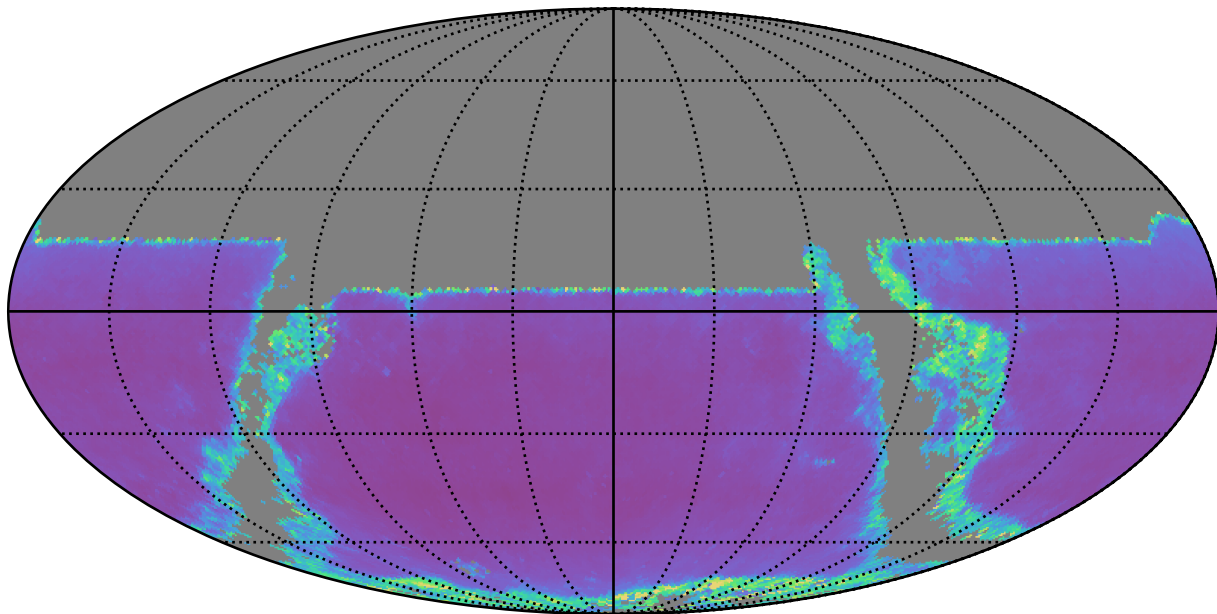
no_long_v3.4_10yrs y band: AGN SF_uncert
